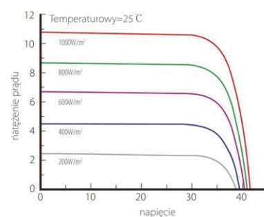
Krzywa prądowo-napięciowa
